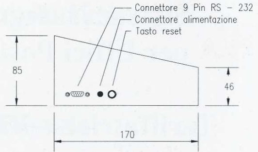
LATERALE
